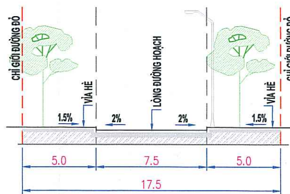
MẶT CẮT 1--1
